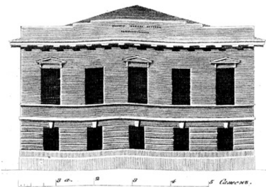
«Собрание фасадов...» 1812 г. Часть 3. Л. 23. Проект фасада, в соответствии с которым разработан фасад «Дома Успенской церкви» в Воронеже
