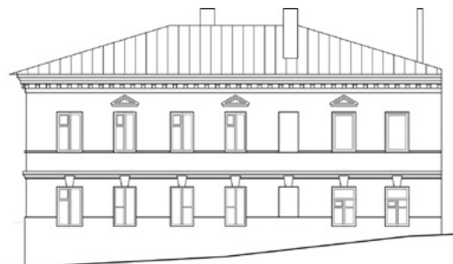
Фасад «Здания Ремесленной управы» в Воронеже. Чертеж А. Кузнецовой, 2018 г.
