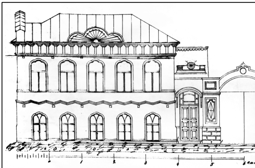
Дом купца В.К. Попова. Проект 1877 г. (ГАВО. Ф. И-19. Оп. 1. Д. 1031. Л. 18 об.)
